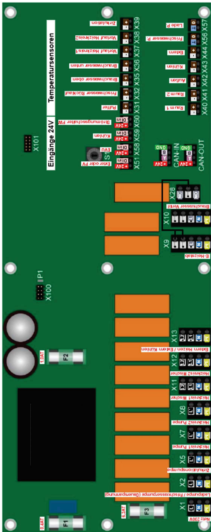
Abbildung 19: Anschlussklemmen AHC Hydraulikregler
