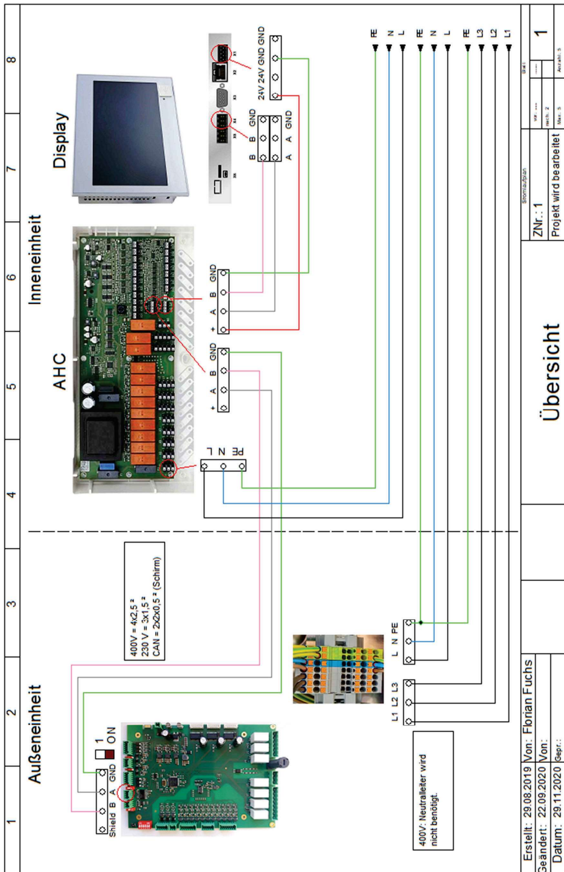
Abbildung 16: Übersicht Verkabelung
